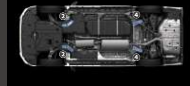
GRブレース装着イメージ(ターボガソリン車・2WD)
