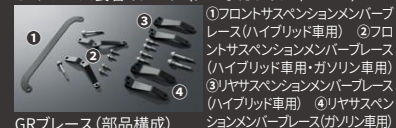
GRブレース(部品構成)
