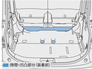
隙間・凹凸部分 (装着前)
