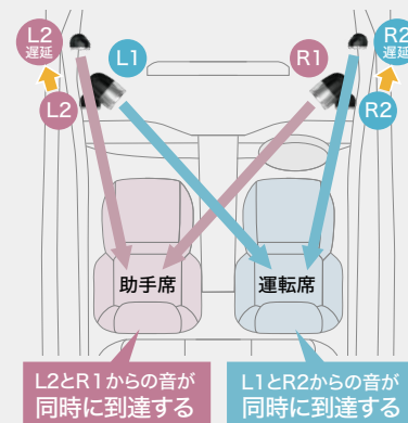
左右席同時定位原理図
