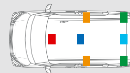
LEDルームランプ配置図
