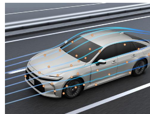
機能あり状態のイメージ: 走行によるタイヤ周りの帯電を低減することで、タイヤ周りの流れの乱れを低減
