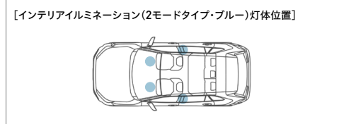
[インテリアイルミネーション(2モードタイプ・ブルー)灯体位置]
